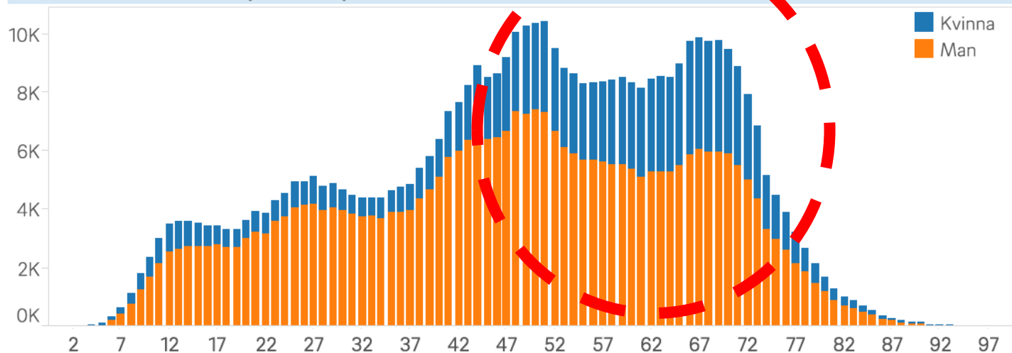
Åldersstrukturen 2015 (individer)
